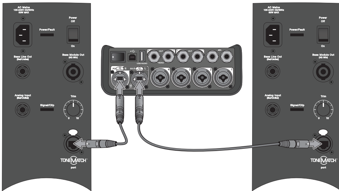
Figura 9 Due sistemi L1 Model II collegati a un mixer T4S tramite connessione digitale
