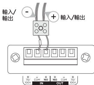
16Ω / 8Ω
