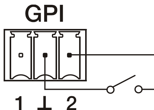
Figure 1 : exemple de connexion du port GPI 2
