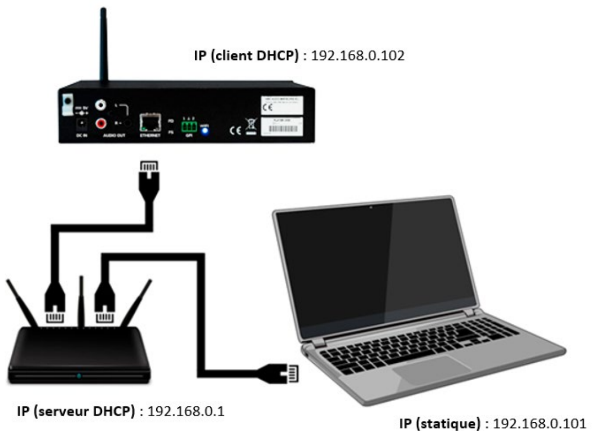
Figure 2 : exemple de connexion à un réseau local par l'interface réseau Ethernet (filaire).
