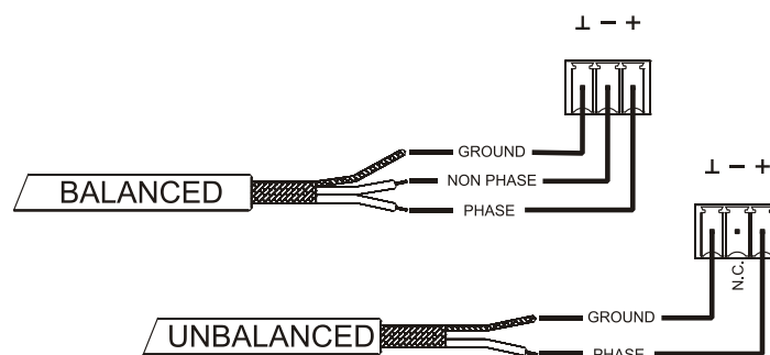
Figure 10 : connexion de sortie audio symétrique
